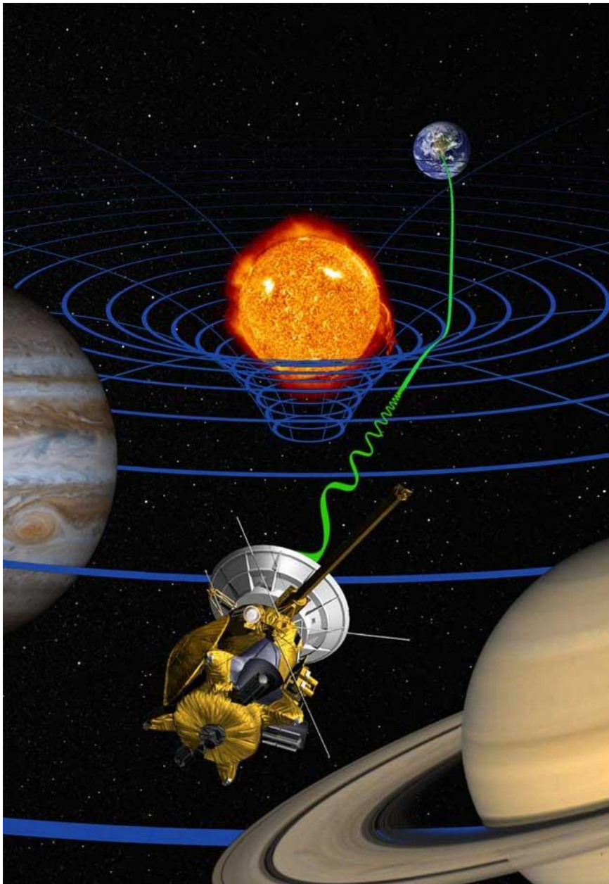
Test de haute précision de la relativité générale par la sonde spatiale Cassini (vue d'artiste) : des signaux radio envoyés entre la Terre et la sonde (onde verte) sont retardés par la déformation de l'espace et du temps due à la masse du Soleil .
